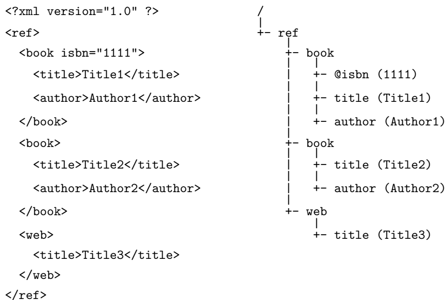
図 1: XSLT における XML 文書のデータモデル (ノード表現)。右側の木において、/ はルートノードであり、@ で始まるノードは属性ノード、その他は要素ノードである。( ) 内は当該ノードの文字列値である。文字列値については後述する。
