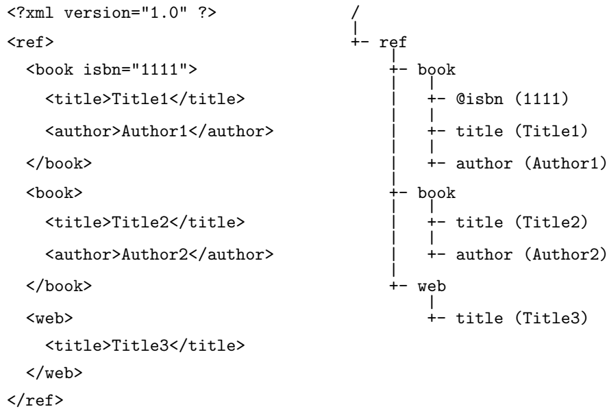
図 1: XSLT における XML 文書のデータモデル (ノード表現)。右側の木において、/ はルートノードであり、その他は要素ノードまたは属性ノードである。ただし、属性ノード名の @ は属性であることが分かるように便宜的に付したものであり、名前の一部ではない。また、( ) 内は当該ノードの文字列値である。文字列値については後述する。
